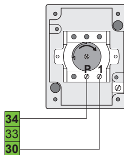
tlačítko chodec (např. klíčový spínač EPZ 1-1T)
